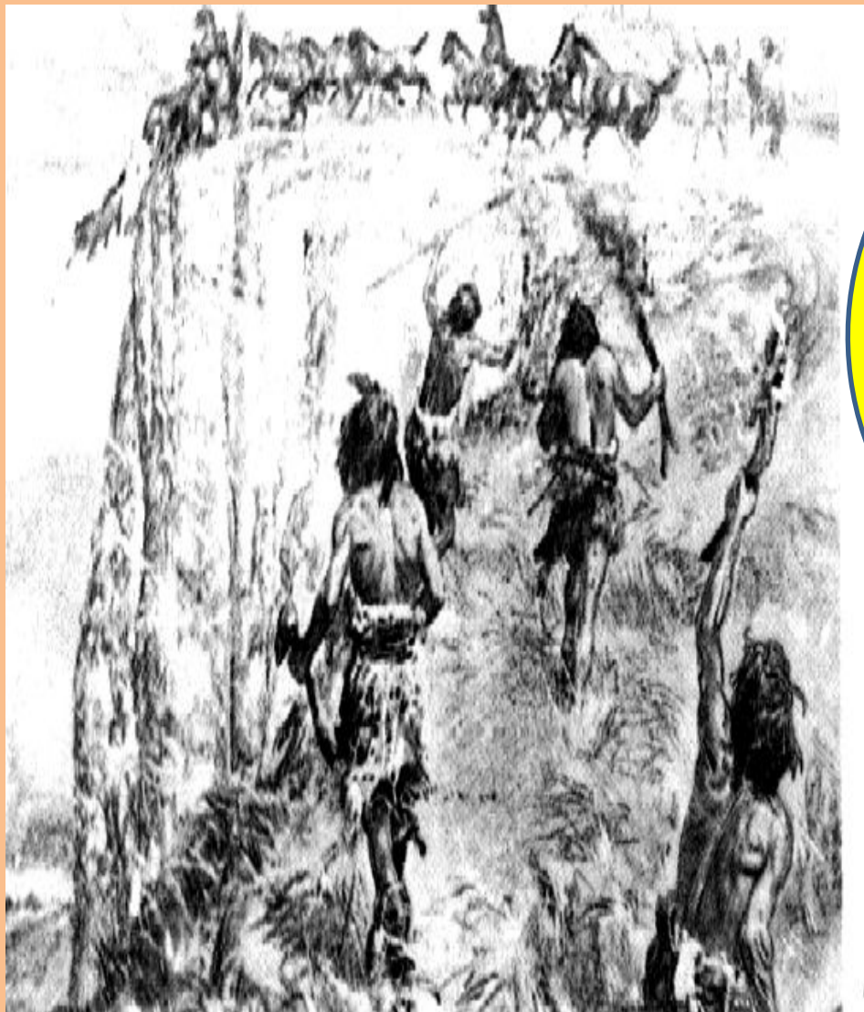
Загонная охота
