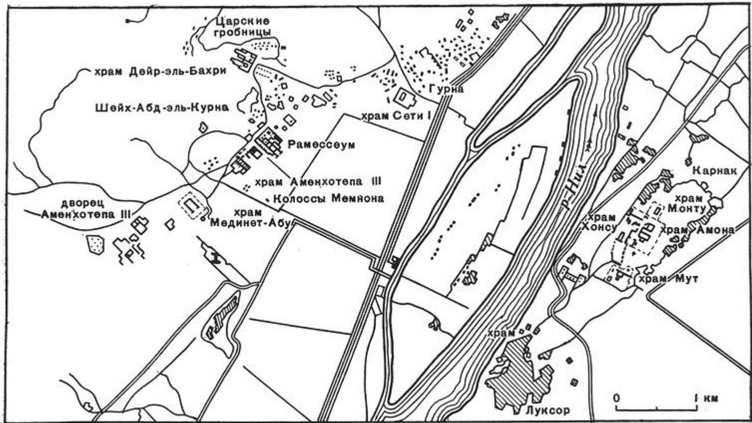
Ансамбль Фив. Генеральный план
