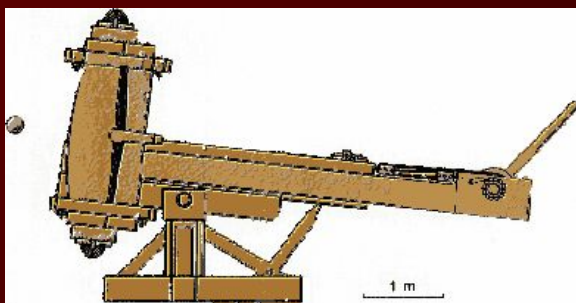
Легионная баллиста
