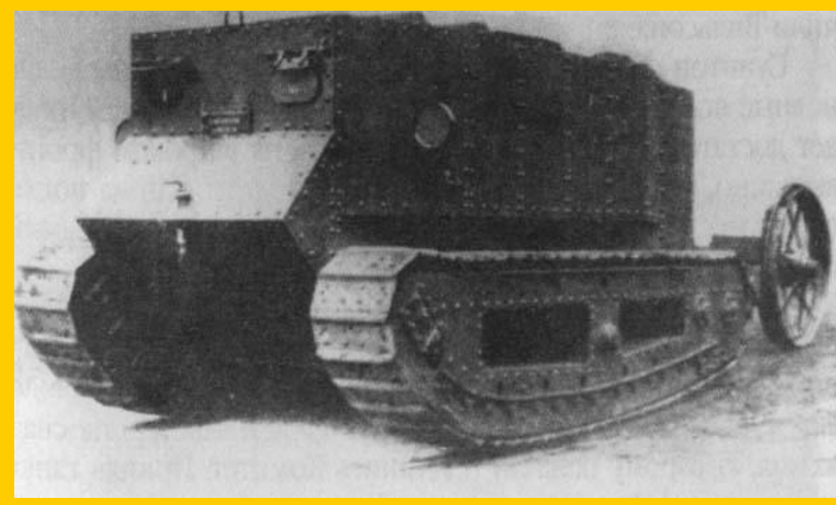
Первый тяжёлый английский танк 1915 г.
