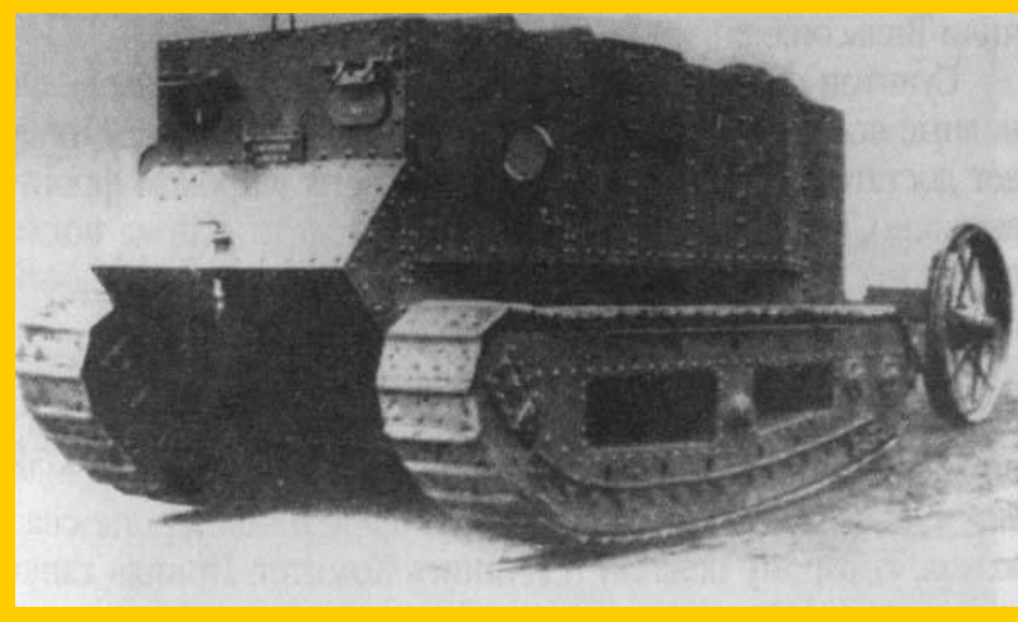
Первый тяжёлый английский танк 1915 г.
