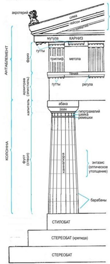
Дорический ордер
