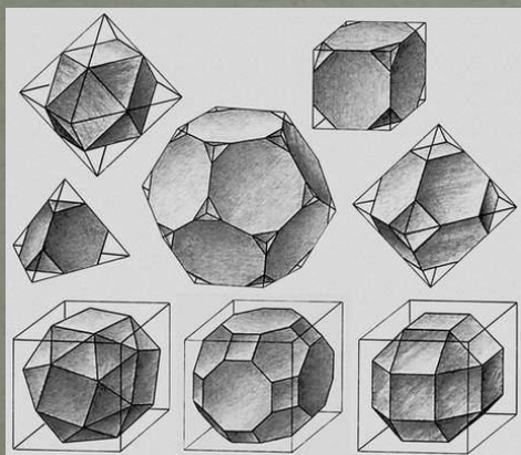
Тела Архимеда
