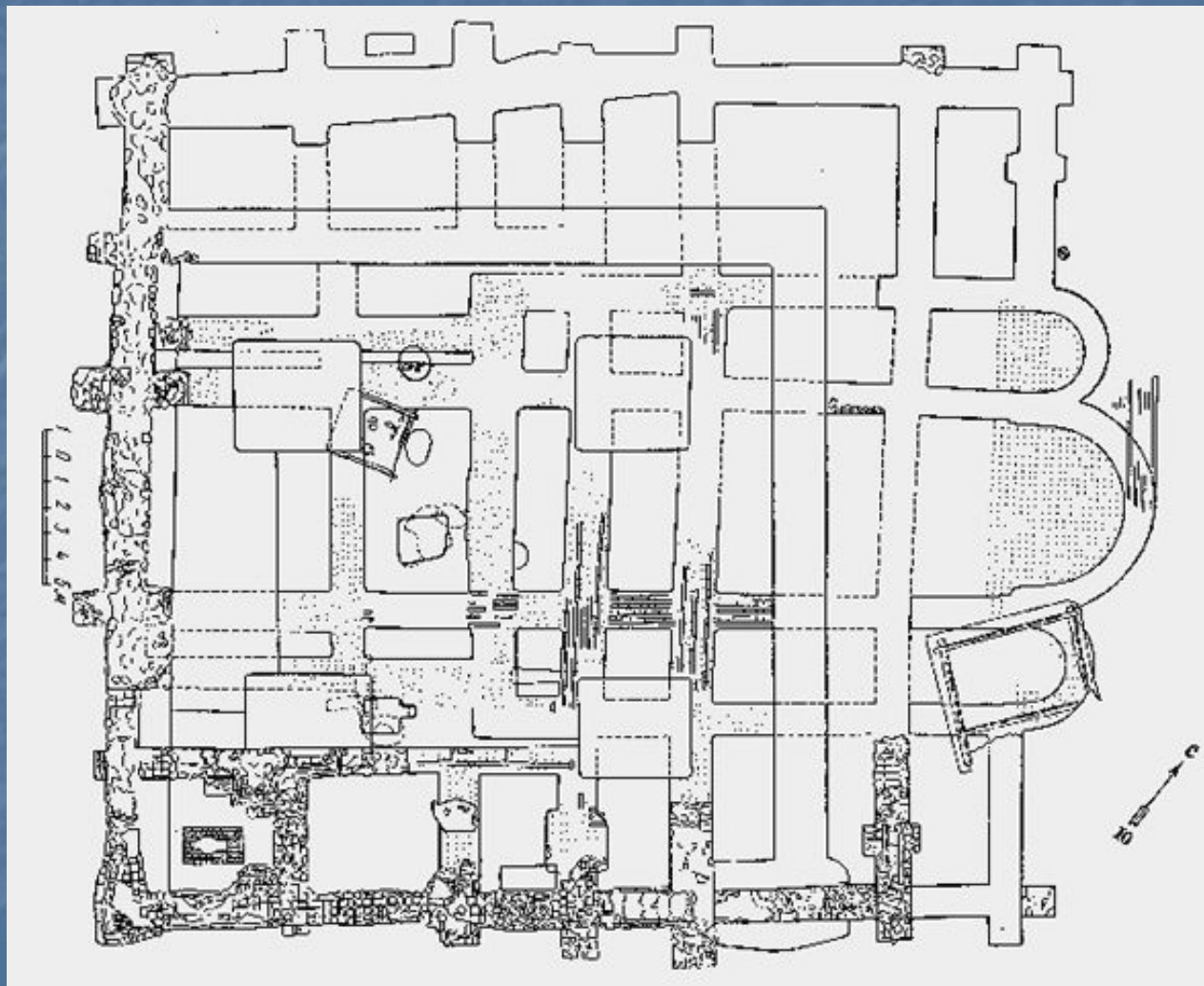
Десятинная церковь в Киеве (план)
