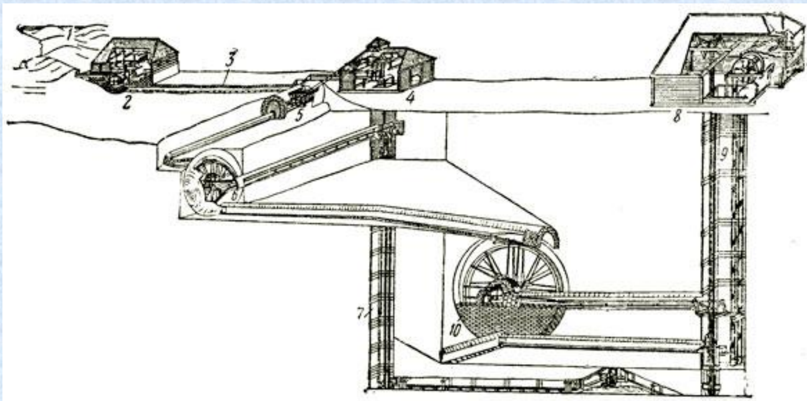
Гидросиловая установка К. Д. Фролова: 1. Плотина; 2. Пильная мельница; 3. Канал; 4. Здание рудоподъёмника Екатеринославской шахты; 5. Кунштшат Екатеринославской шахты; 6. Кунштшат Екатеринославского водоподъёмника; 7. Екатеринославская шахта; 8. Надшахтный сарай Вознесенской шахты; 9. Вознесенская шахта; 10. Кунштшат Вознесенского рудо-водоподъёмника
