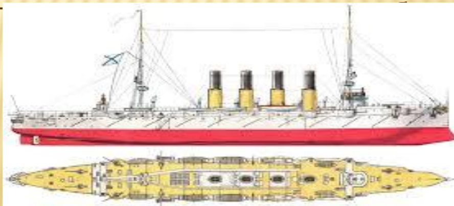
Российский крейсер 1 ранга "Варяг". Слева: вид сверху, справа: вид сбоку.
