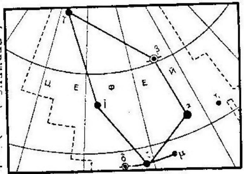
Созвездие Цефея
