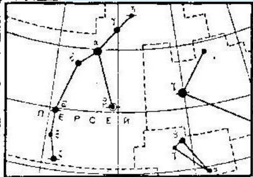
Созвездие Персея
