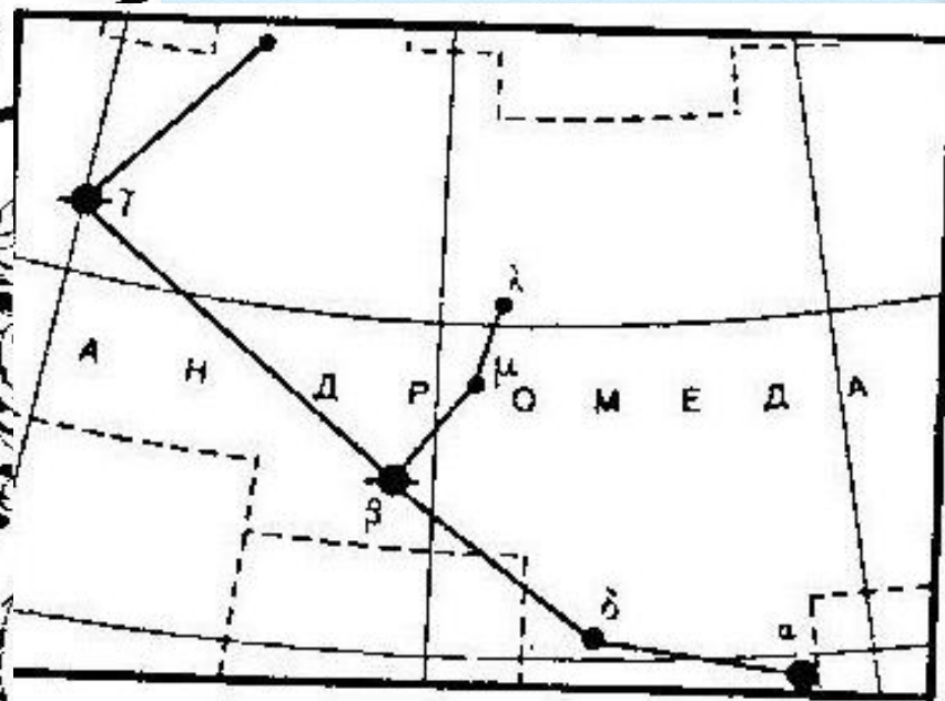
Созвездие Андромеды
