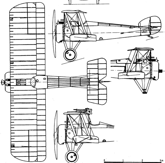
Sopwith F. 1 CAMEL
