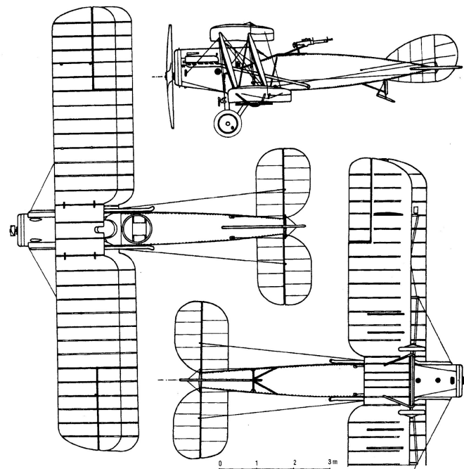
Bristol F. 2B
