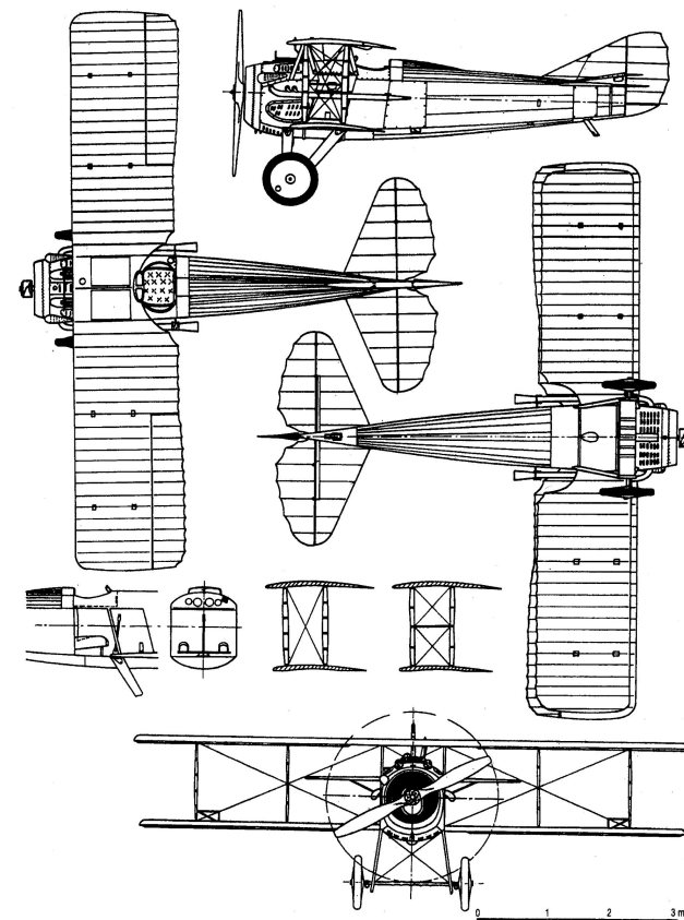
SPAD S.13Ca
