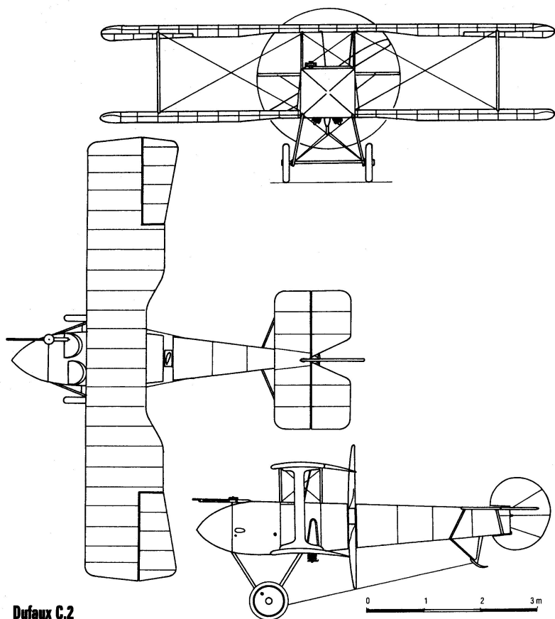
Dufaux C.2
