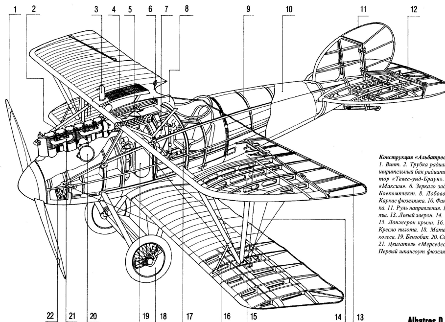
Albatros D.V
