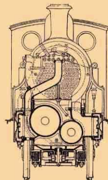
Черт. 6. Коммунальный паровоз Ворделла (Worsdell).
