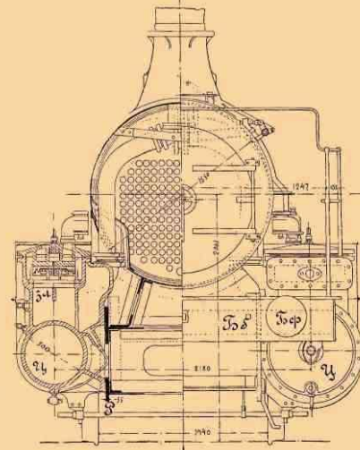
Черт. 6. Коммунальный паровоз Ворделла (Worsdell).
