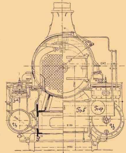
Черт. 6. Компа угле-паровоз Воределя (Worsdell).
