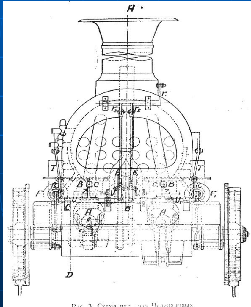
Рис. 3. Схема паровоза Черепановых.
