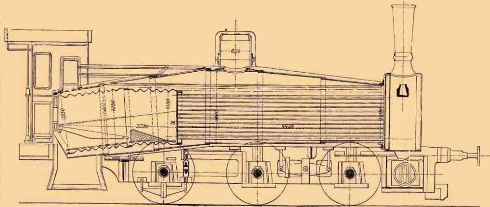
Черт. 5. Товарный паровоз с котлом Ленца (Lentz).
