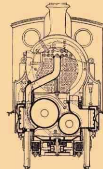
Черт. 6. Коммунальный паровоз Воредела (Worsdell).
