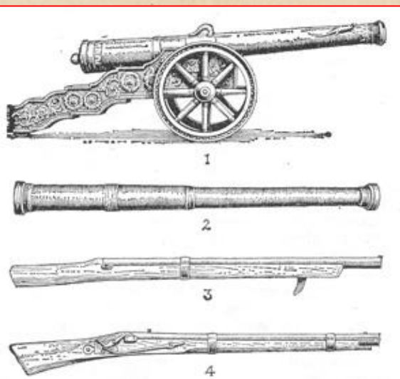
Пищали: 1 — осадная на декоративном лафете 16 в.; 2 — бронзовая конца 15 в.; 3 — «затинная» (крепостная) сер. 16 в.; 4 — «завесная» (носившаяся за плечом на ремне) с фитильным замком конца 16 в.
