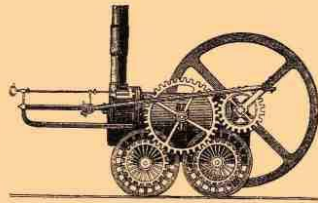
2. Паровоз Тревитика (1804).
