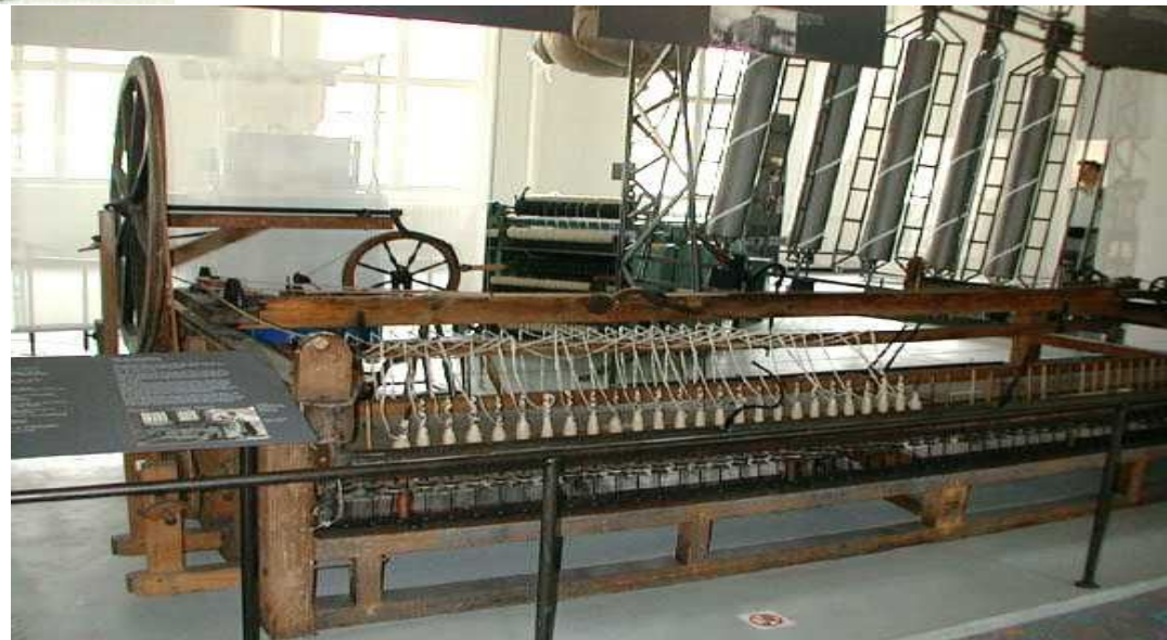
Прядильная машина «Дженни» Дж. Харгривса
