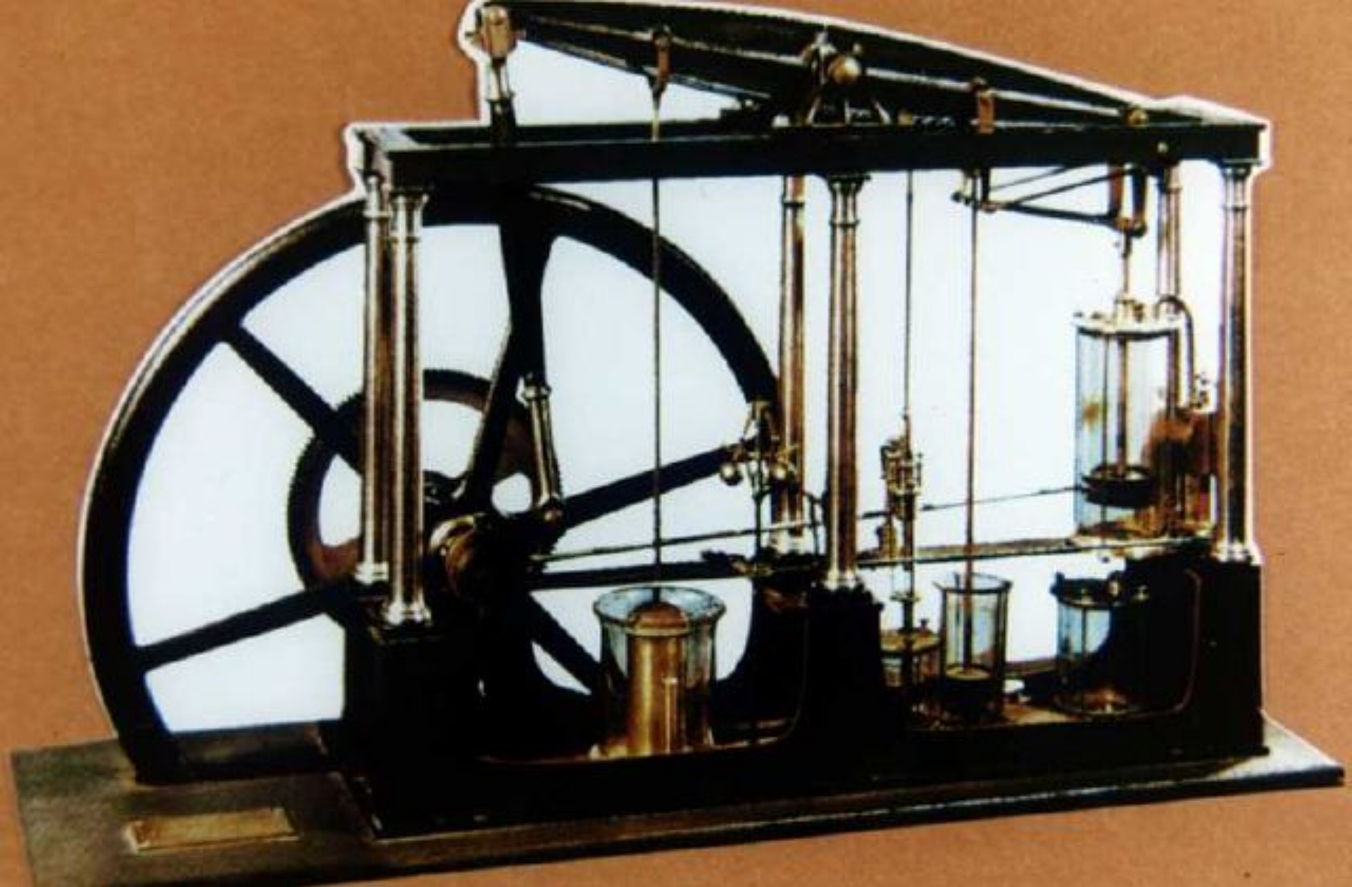
Паровая машина, созданная Дж. Уаттом
