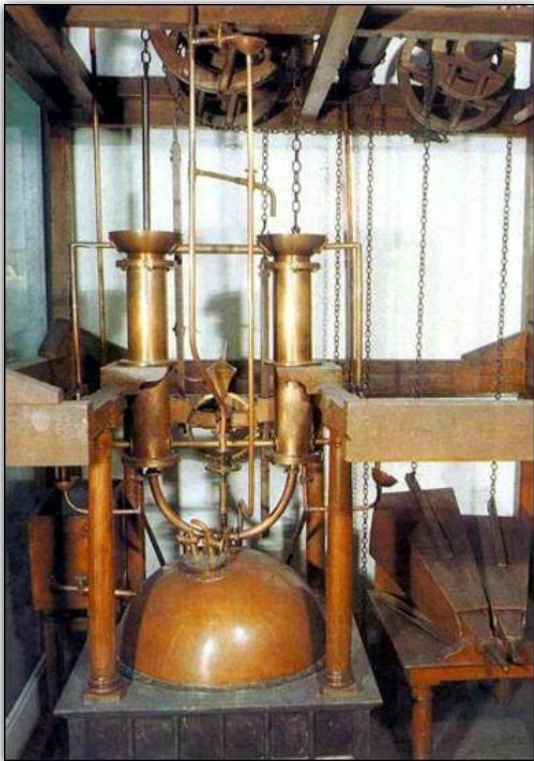
Паровая машина Ползунова
