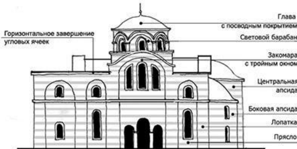
Фасад византийского храма
