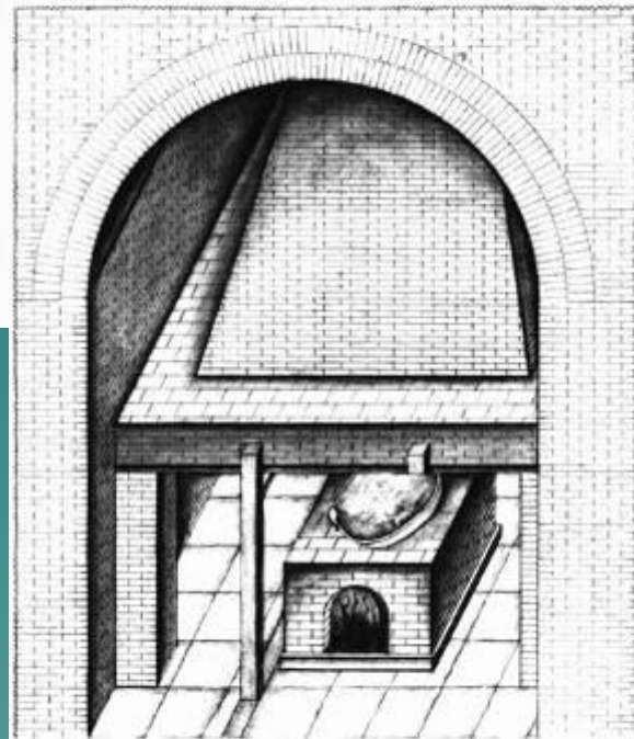
Л. Отбильная печь.
