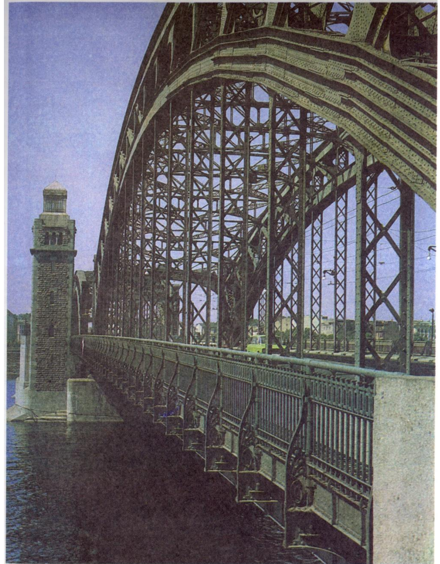
Большеохтинский мост, Санкт-Петербург (1911), инженер Г. Кривошеин и архитектор В. Альшков
