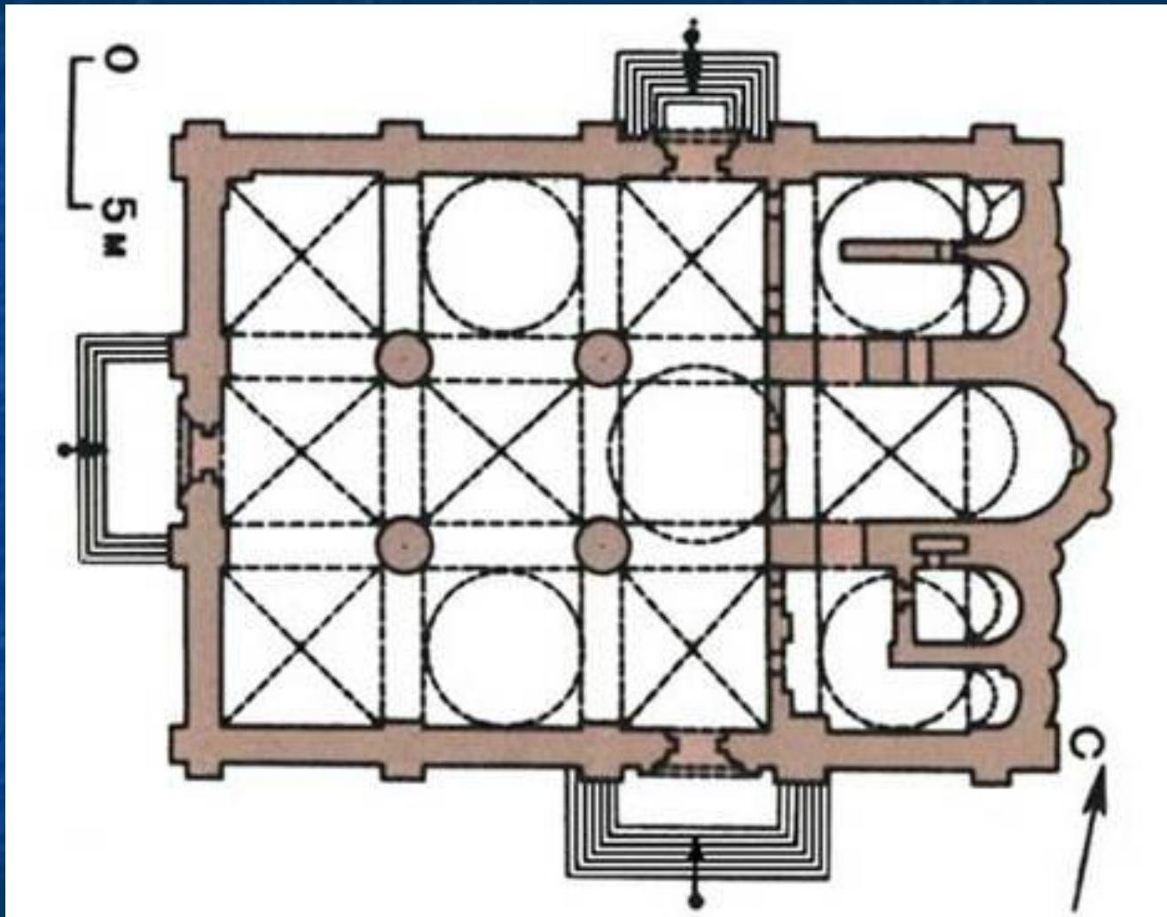
Аристотель Фиораванти. Успенский собор Московского Кремля. 1497 г. План
