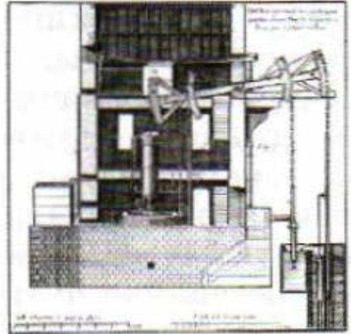
Паровая машина Ньюкомена для откачки воды. Гравюра из книги Белидора «Гидравлические сооружения». XVIII в.
