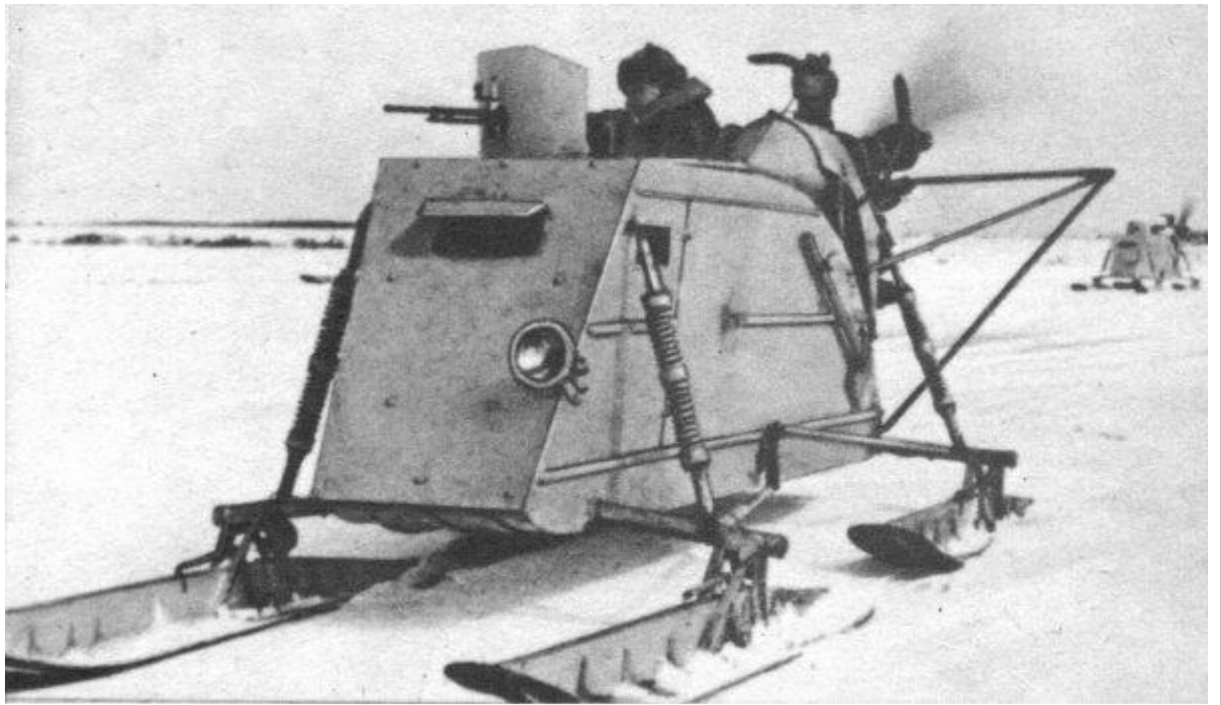
Аэросани времен ВОВ
