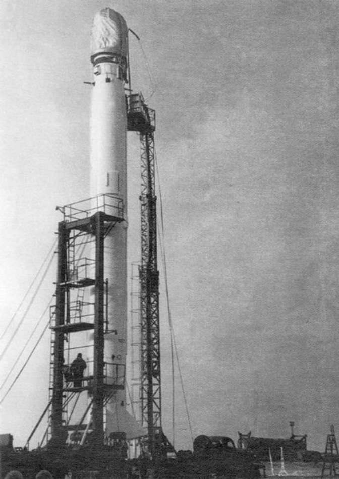
Ракета средней дальности Р-5М. Принята на вооружение в 1956 г. Первая советская ракета, способная нести ядерное оружие.
