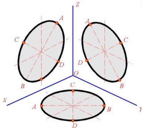
Изометрическая проекция
