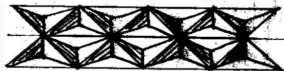
Элемент "Розетка"
