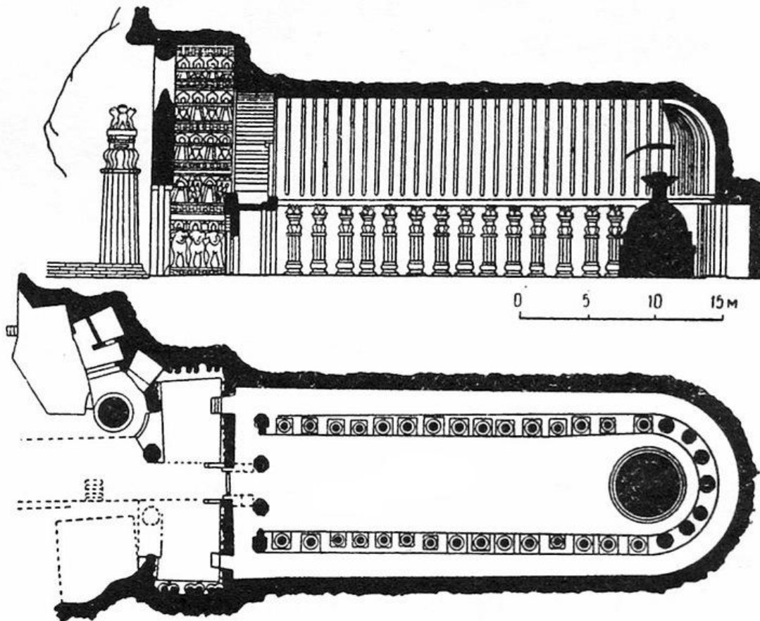
Карли. Буддийский храм — чайтья, I в. до н. э. Общий вид, интерьер, продольный разрез, план
