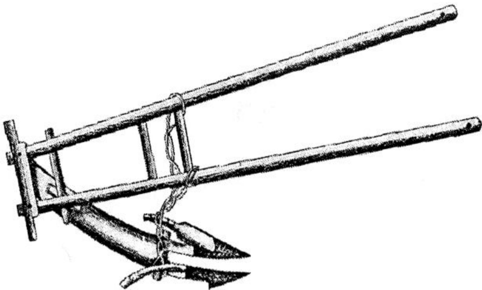
3. Соха с перекладной полицей. Рисунок А.И.Гильденштедта (Технологический журнал, т. I, ч. II, СПб., 1804. Приложения).
