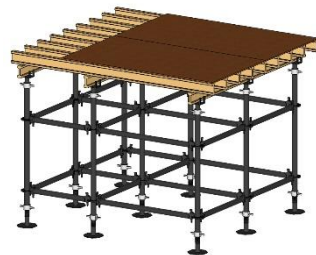
Объемная опалубка
