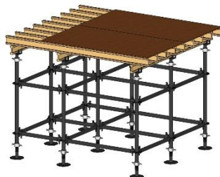
Объемная опалубка
