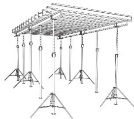
Опалубка перекрытий
