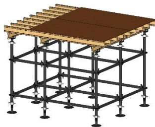
Опалубка перекрытий
