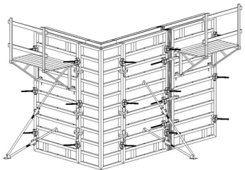
Стеновая опалубка
