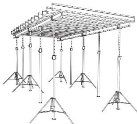
Опалубка перекрытий
