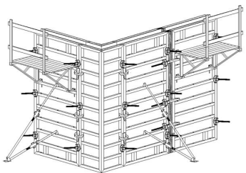
Стеновая опалубка
