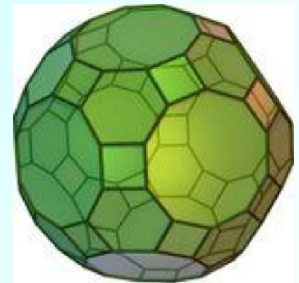
Ромбоусеченный икосододекаэдр
