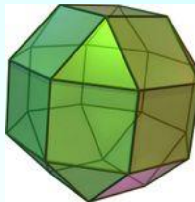
Ромбокубооктаэд р
