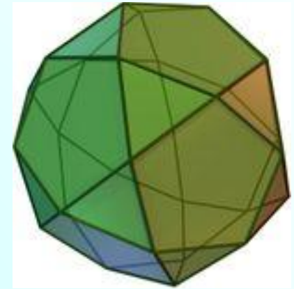
Икосододекаэдр
