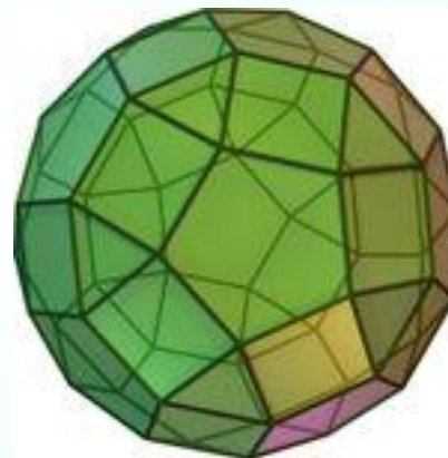
Ромбоикосоододекаэд р
