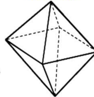
октаэдр
