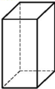
прямоугольный параллелепипед
