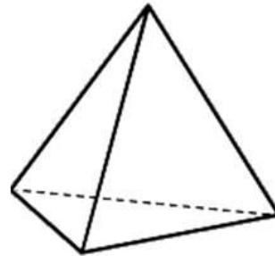
тетраэдр
