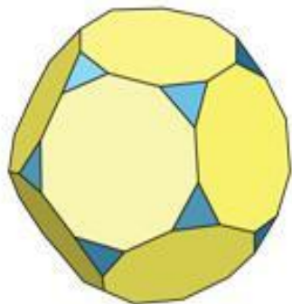
усечённый додекаэдр
