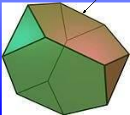
Усечённый тетраэдр
