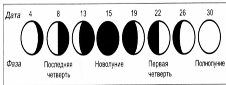
Фазы Луны
