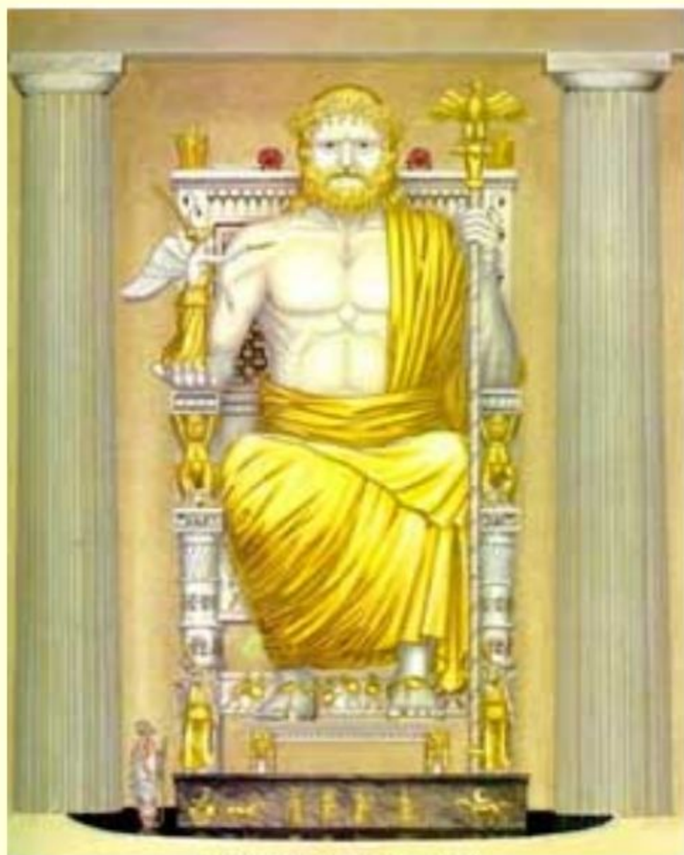
Статуя Зевса
