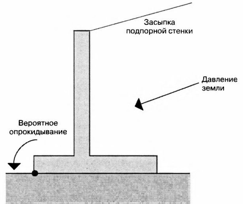
Рис. 6.6. Подпорная стенка, установленная на камень
