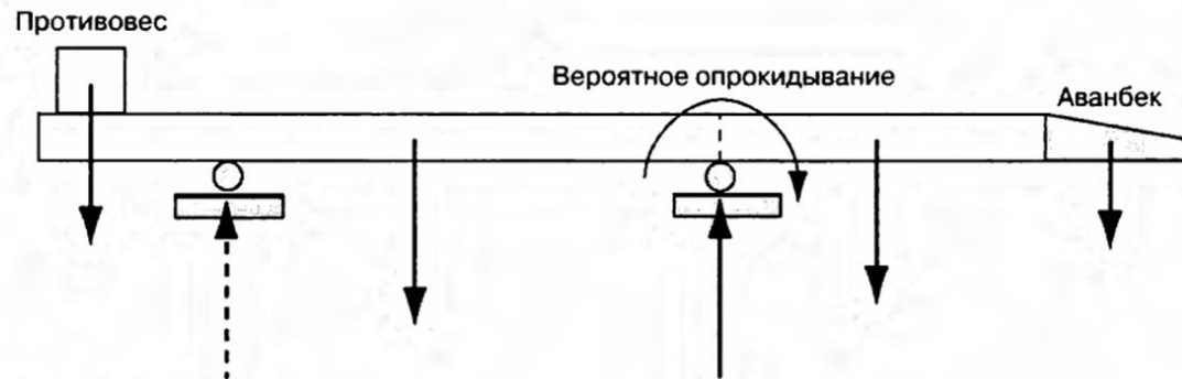
Рис. 6.5. Пример наведения настила моста
