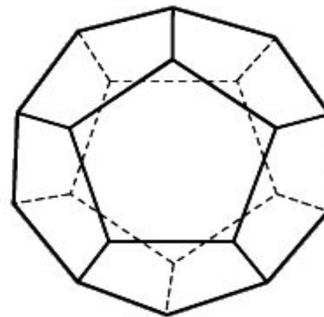
Додекаэдр
