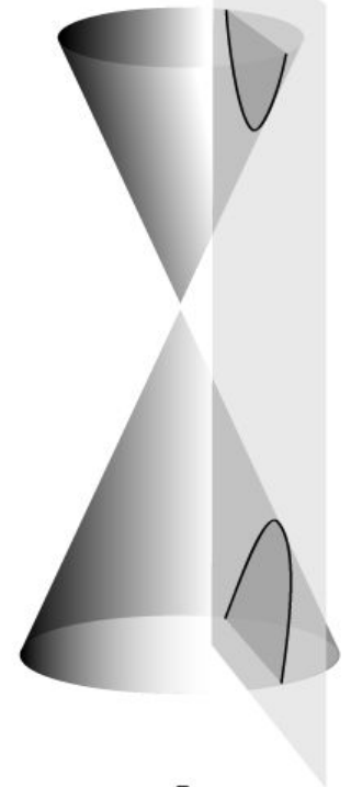
Гипербола
