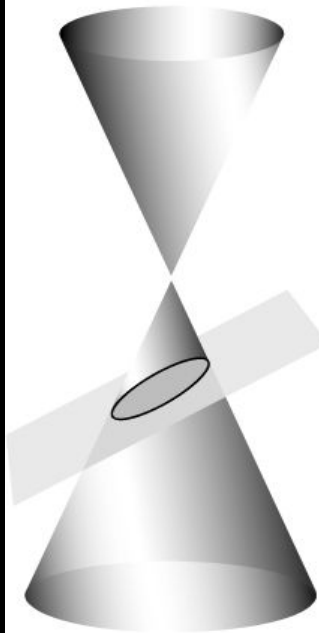
Эллипс
