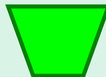
четырёхугольники
