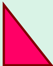
треугольники
