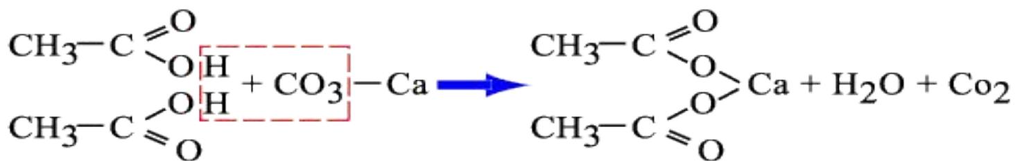
уксусная кислота
