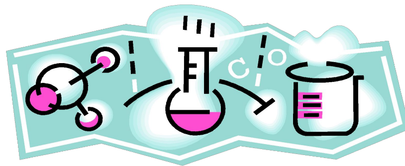
ацетат кальция
