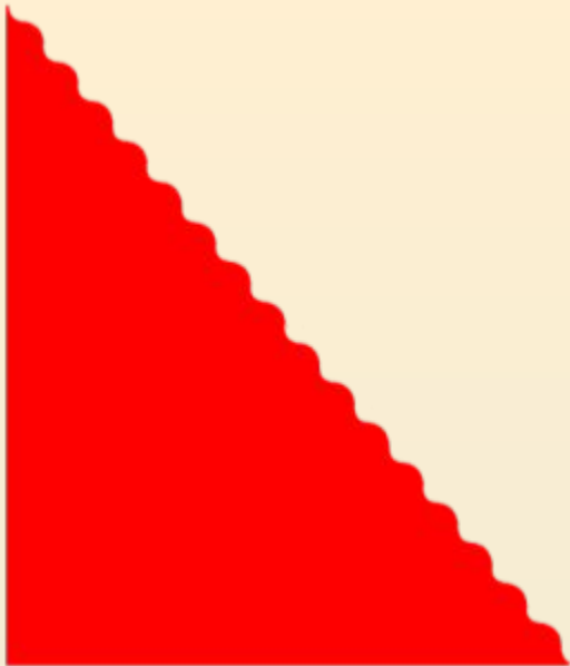
Прямой угол
