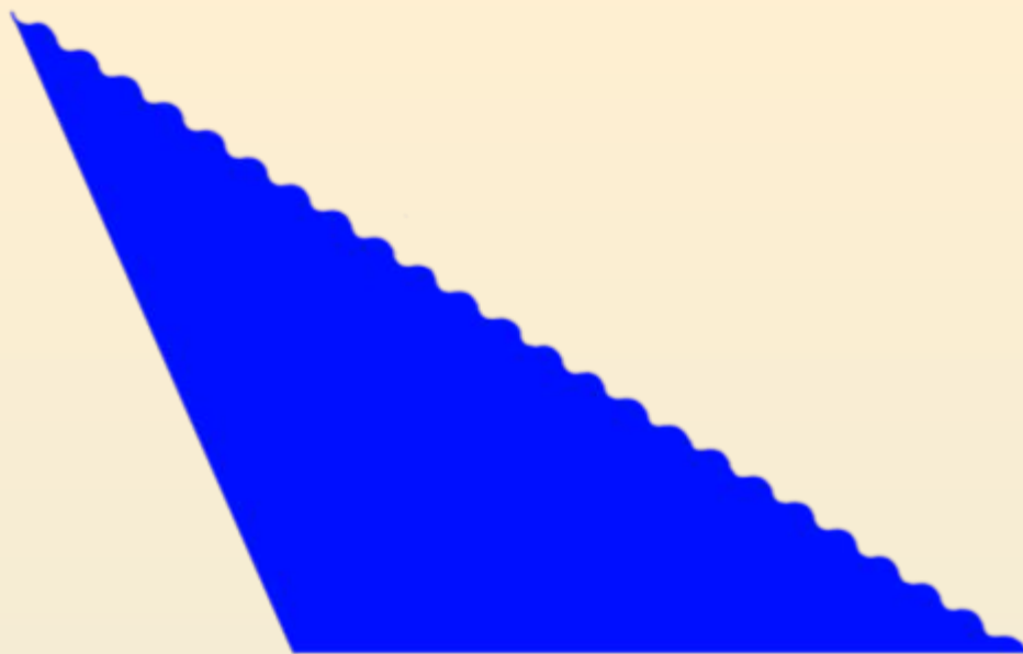
Тупой угол
