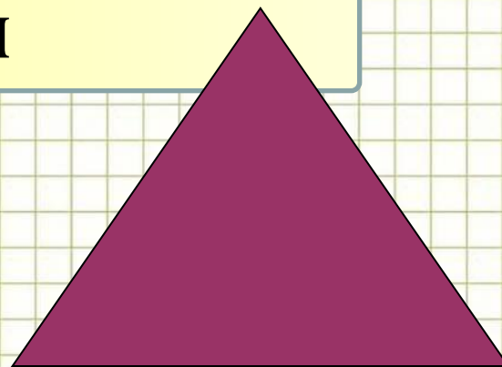
треугольник
