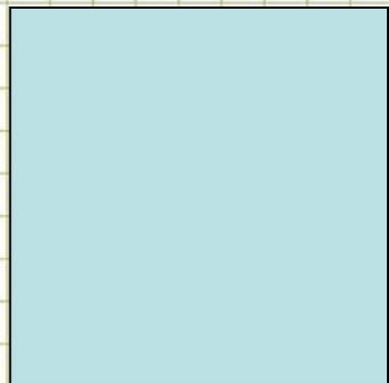
квадрат
