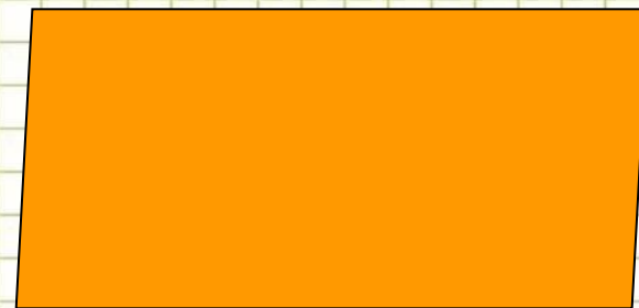
четырёхугольник
