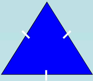
Равносторонний треугольник
