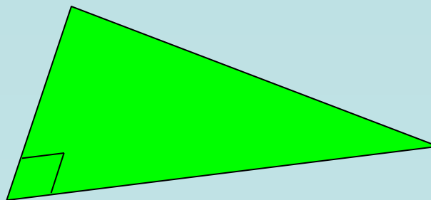
Произвольный треугольник
