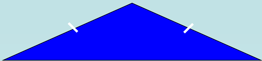
Равнобедренный треугольник
