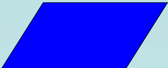
Параллелограмм
