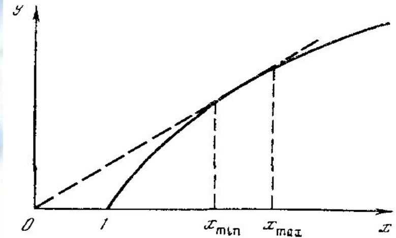
Рис. 17. График логарифмической функции
