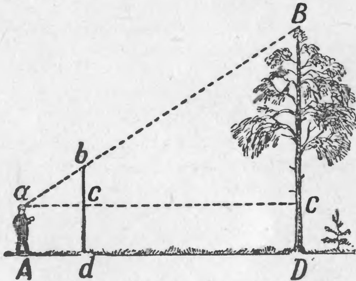
Рис. 8. Измерение высоты дерева при помощи шеста.
