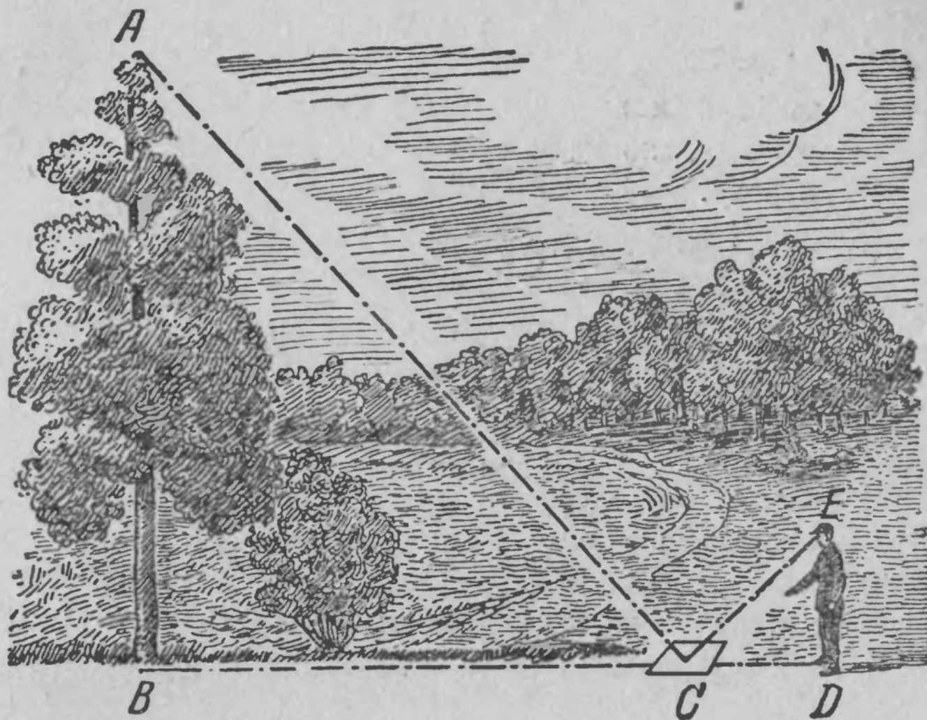
Рис. 14. Измерение высоты при помощи зеркала.
