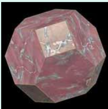
усеченный октаэдр
