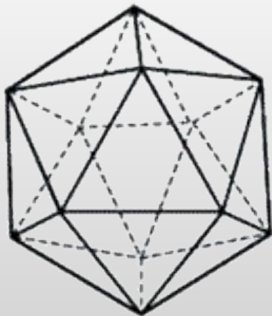
Икосаэдр
