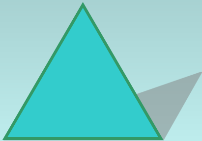
Правильный треугольник
