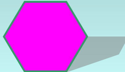
Правильный шестиугольник
