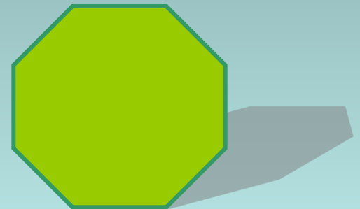
Правильный восьмиугольник
