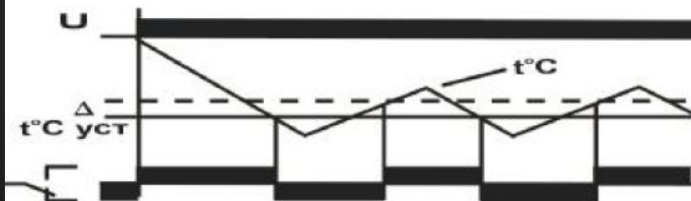
Режим «охлаждение»
