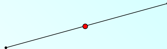
Отрезок
