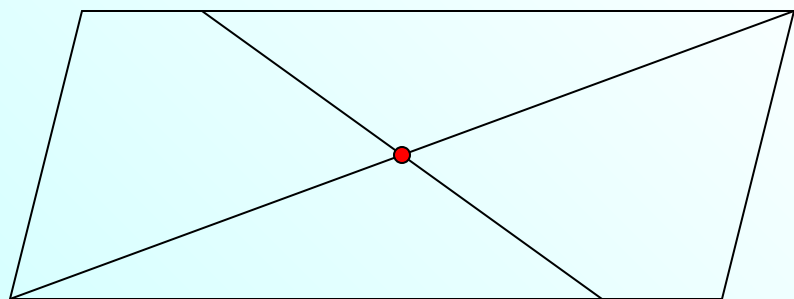
Параллелограмм
