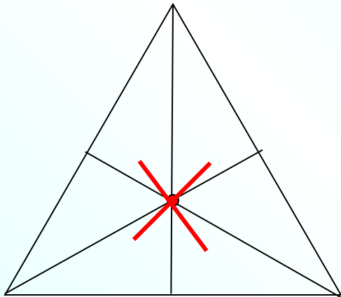
Правильный треугольник
