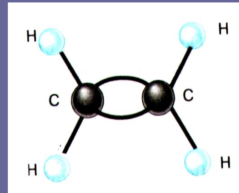
Молекула этилена
