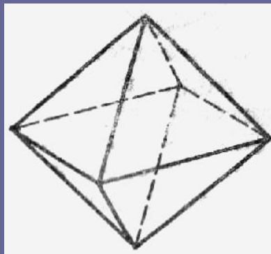
Октаэдр
